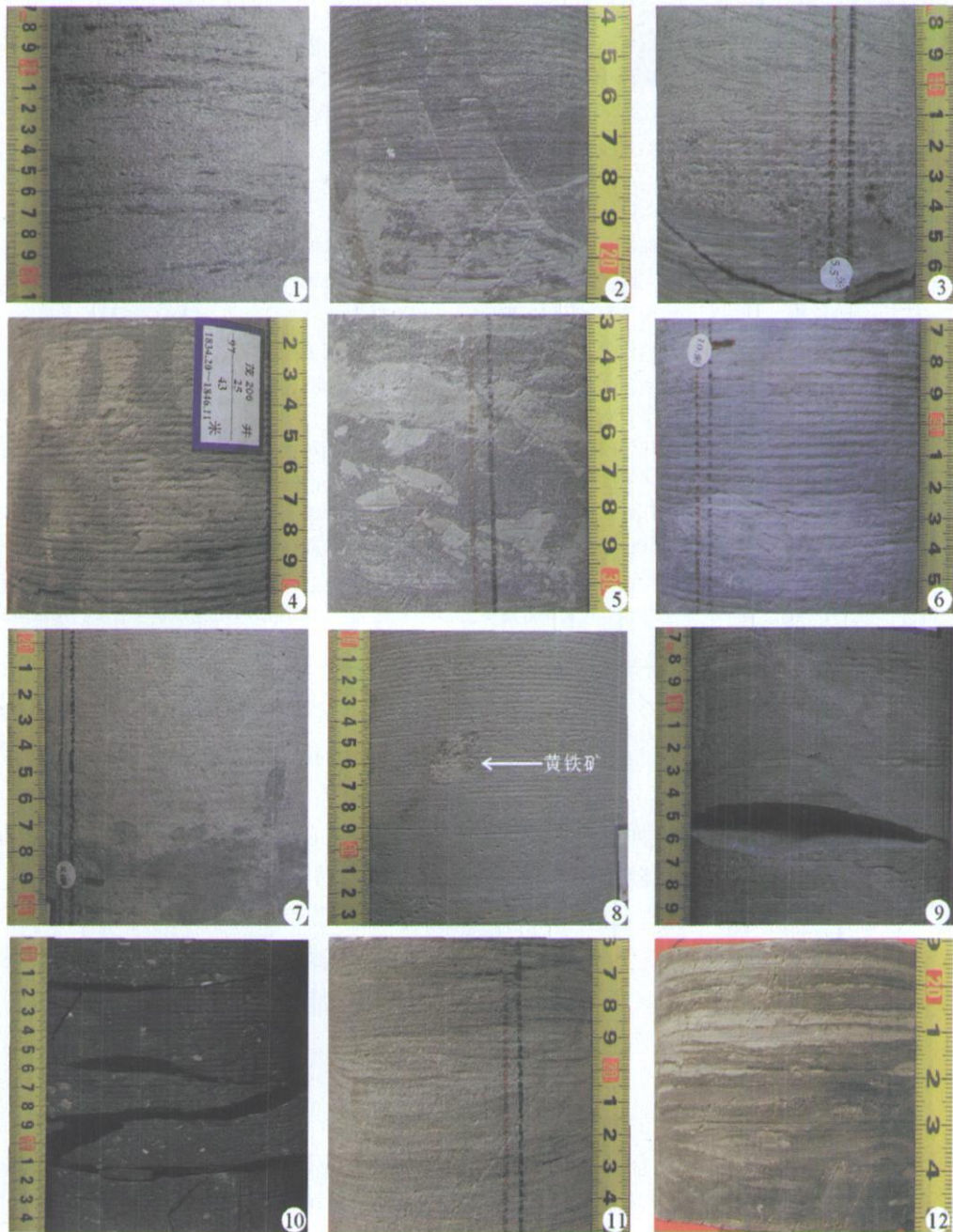
图版 I 松科 1 井南孔泉头组岩性、沉积相特征图版
