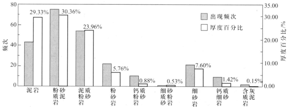
图2 松科1井南孔泉头组岩心岩性出现频次、厚度百分比图
